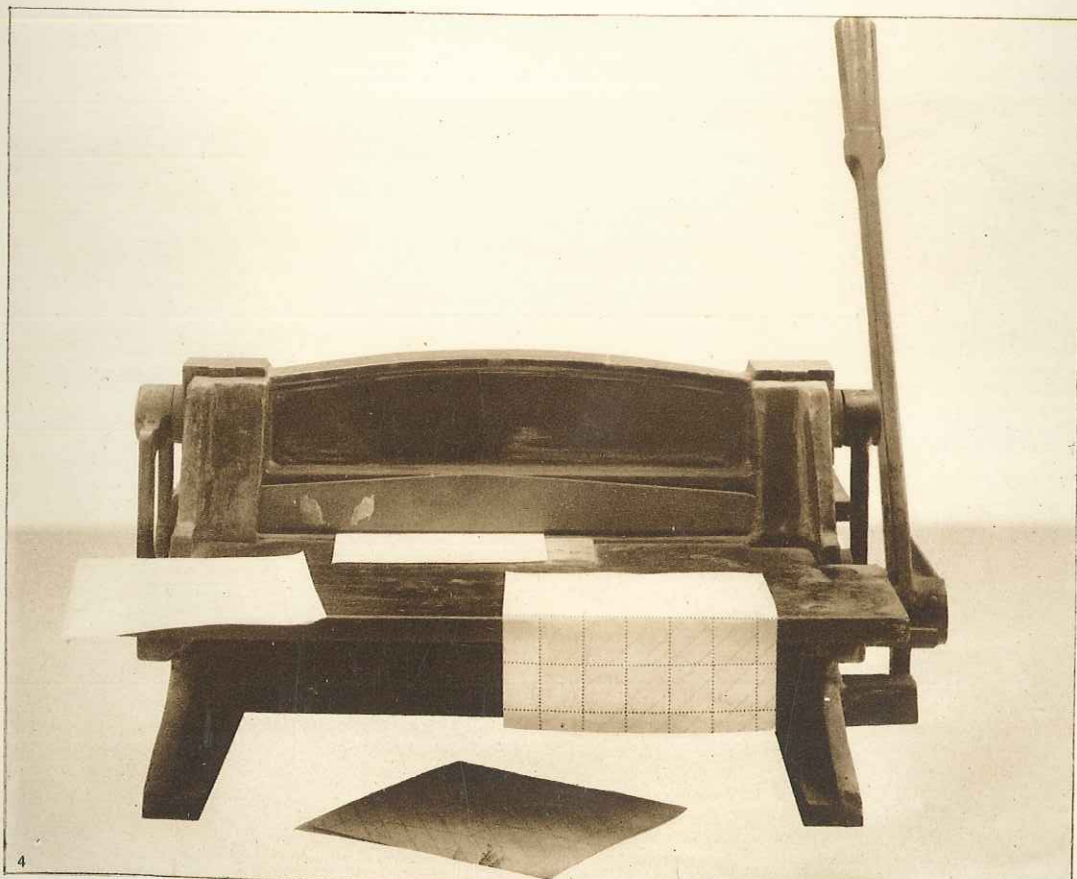
Machine à denteler les timbres.
