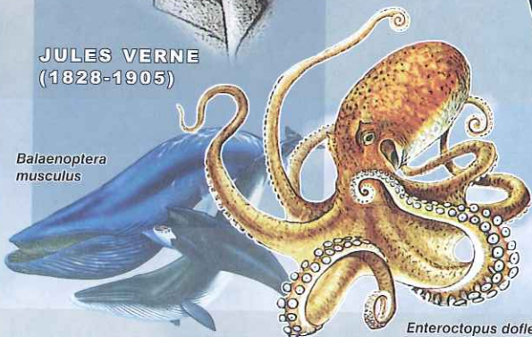
Enteroctopus doffeini
