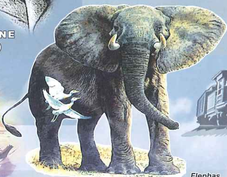
Elephas
