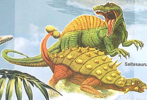
Ankylosaurus
