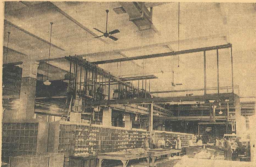
Palacio de Correos y Telégrafos. — Un aspecto de las instalaciones electromecánicas para el transporte interno de la correspondencia. Buenos Aires. — República Argentina.
